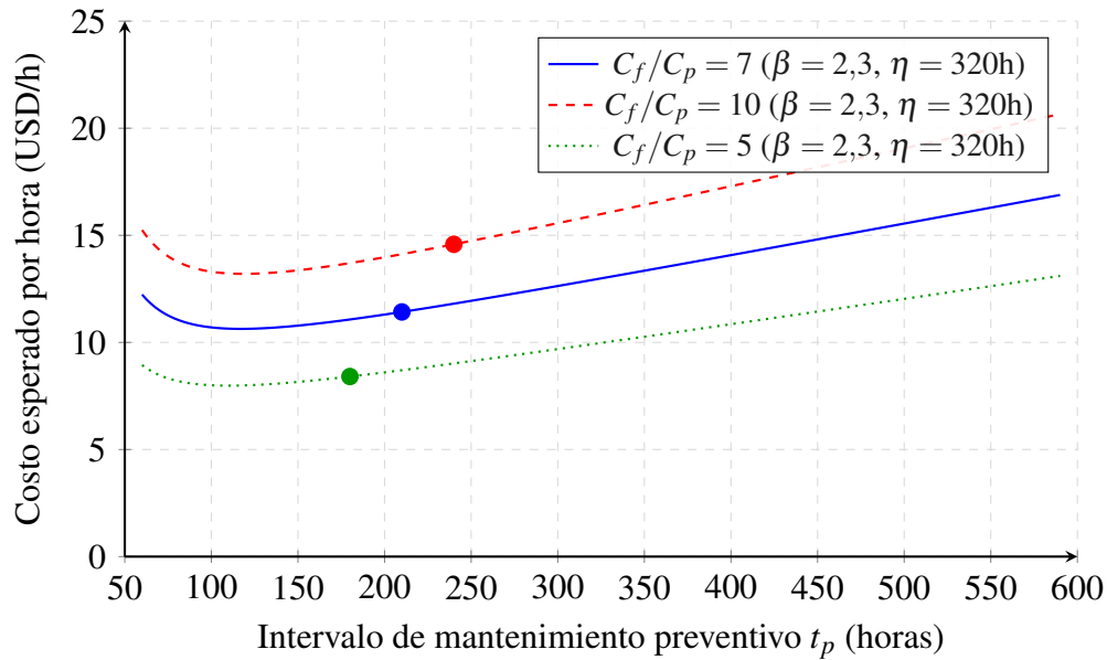
Figura 10: Sensibilidad del costo de mantenimiento al intervalo t_p para distintas razones C_f/C_p .
