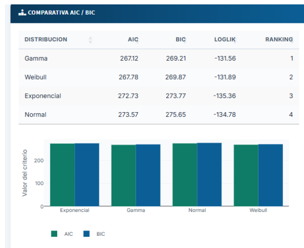
Figura 11: Comparativa de criterios AIC y BIC para la selección del mejor modelo de distribución.
