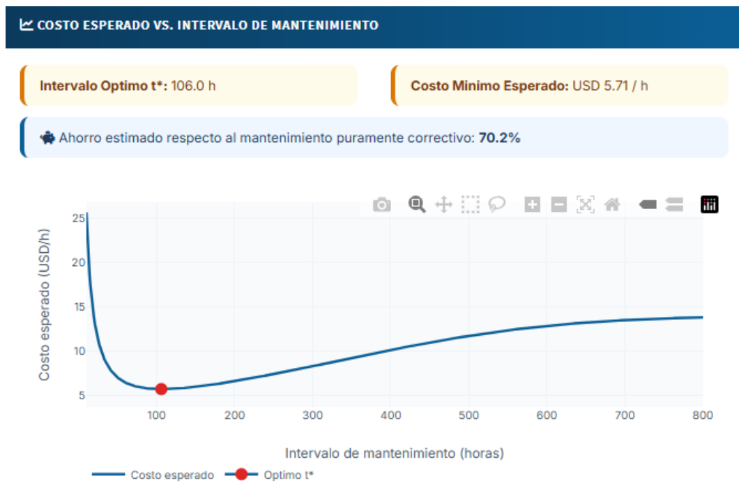
Figura 13: Costo esperado de mantenimiento por unidad de tiempo en función del intervalo t_p .
