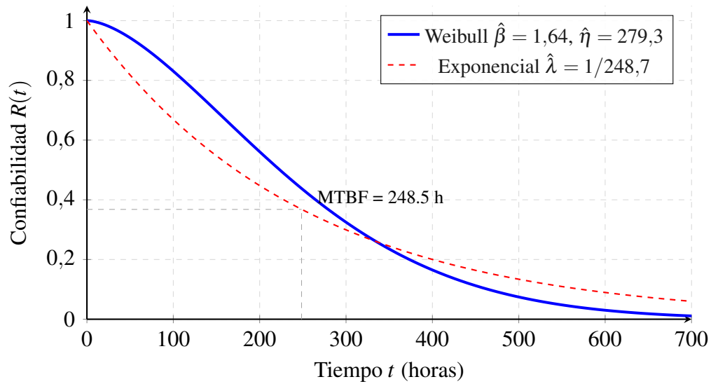
Figura 12: Función de confiabilidad Weibull ajustada vs. Exponencial para el sistema termo-hidráulico.
