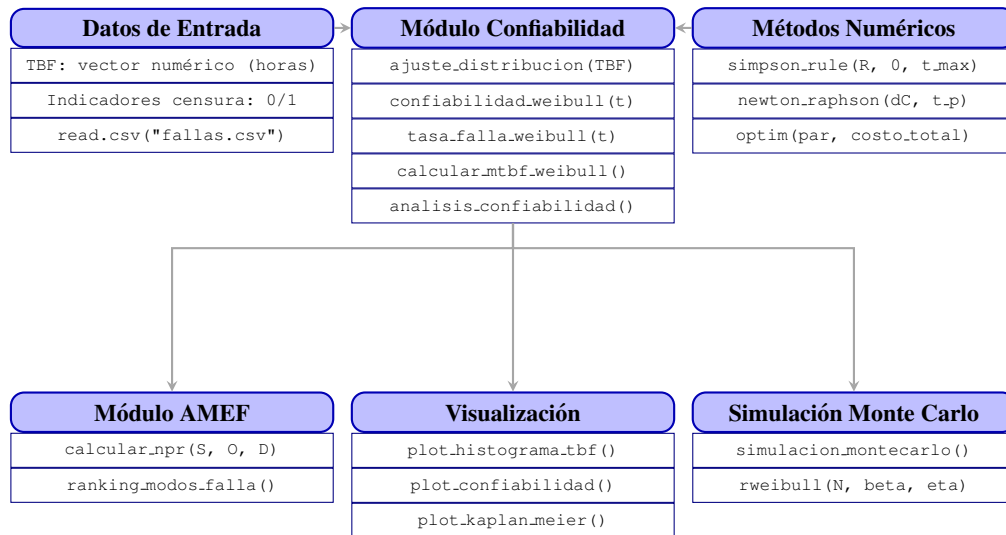
Figura 14: Diagrama de módulos del sistema de análisis de confiabilidad en R.
