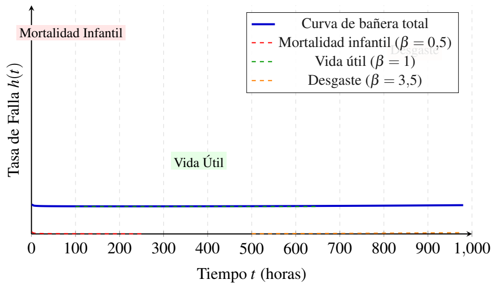
Figura 3: Curva de bañera del sistema termo-hidráulico (combinación de distribuciones Weibull).
